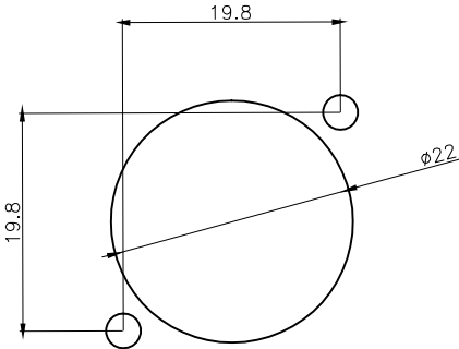
Frontplattenausschnitt (Rueckseite) Panel cut out (rear side)
